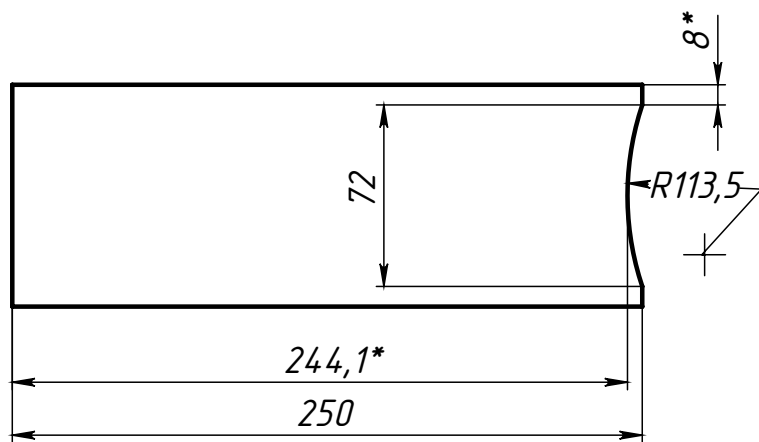
Поз.1 (Основание)
