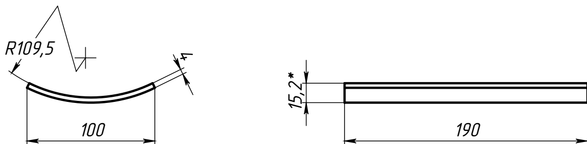
Поз.3 (Ложемент)
